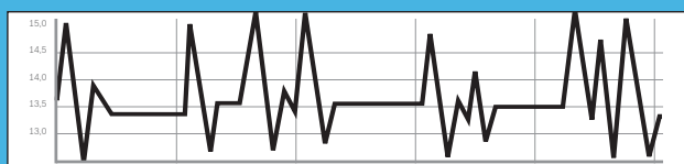
Diagram zaťaženia akumulátora pre systém Štart/Stop a rekuperáciu
