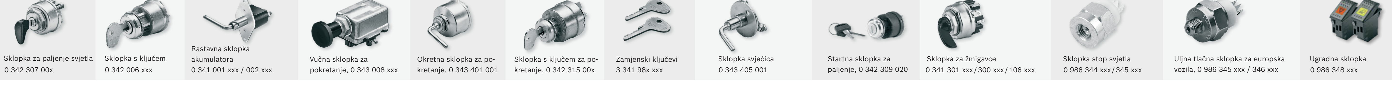
Sklopka za paljenje svjetla 0 342 307 00x Sklopka s ključem 0 342 006 xxx Rastavna sklopka akumulatora 0 341 001 xxx/002 xxx Vučna sklopka za pokretanje, 0 343 008 xxx Okretna sklopka za pokretanje, 0 343 401 001 Sklopka s ključem za pokretanje, 0 342 315 00x Zamjenski ključevi 3 341 98x xxx Sklopka svjećica 0 343 405 001 Startna sklopka za paljenje, 0 342 309 020 Sklopka za žmigavce 0 341 301 xxx/300 xxx/106 xxx Sklopka stop svjetla 0 986 344 xxx/345 xxx Uljna tlačna sklopka za europska vozila, 0 986 345 xxx / 346 xxx Ugradna sklopka 0 986 348 xxx
